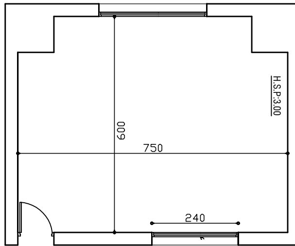
salle existante Institut Supérieur de Sport et de l'Education Physique du Kef
