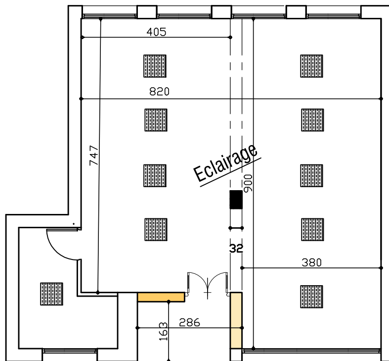
Amenagement d'une salle existante en Salle d'apprentissage actif Institut Sylvio-pastoral de Tabarka
