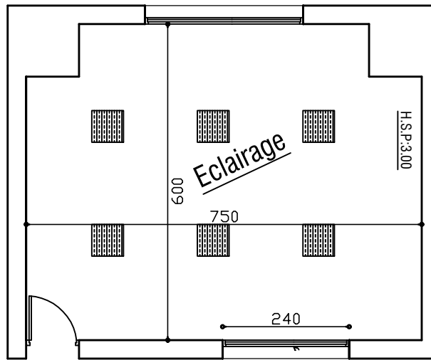
Amenagement d'une salle existante en Salle d'apprentissage actif Institut Supérieur de Sport et de l'Éducation Physique du Kef
