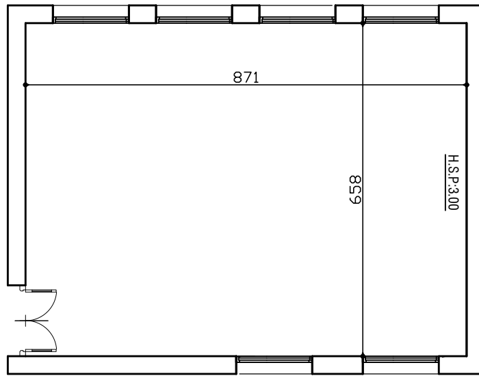
salle existante Institut Supérieur des Sciences Humaines de Jendouba
