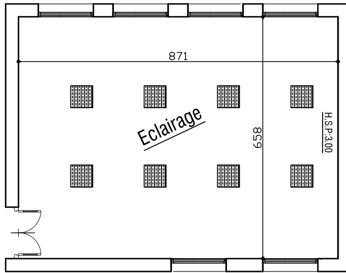
Amenagement d'une salle existante en Salle d'apprentissage actif Institut Supérieur des Sciences Humaines de Jendouba
